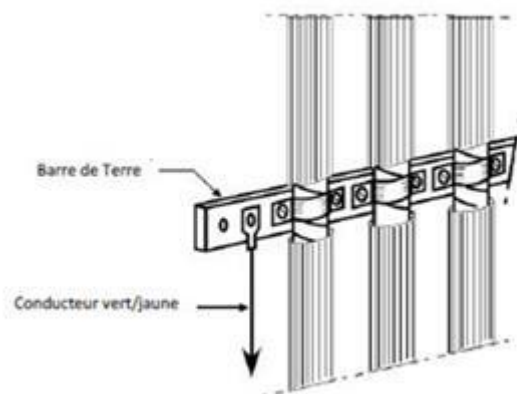
Mise à la terre de câbles écrantés
